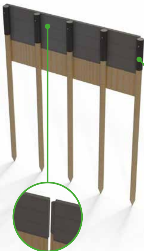
schot met veer/groef verbinding
